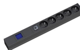
Regleta 5 UTE con monitorización. PDU 5 UTE monitored.
