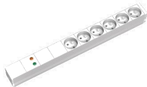
Regleta 6 UTE con PST y filtro. PDU 6 UTE with OVP and filter.
